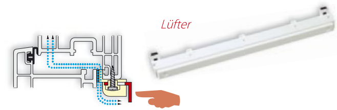
REGEL-air® ÜL - Überschlags-Lüfter für Kunststoff-Fenster
