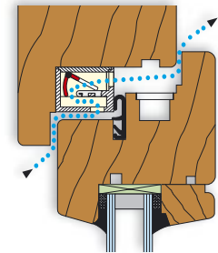
REGEL-air® H - Fensterfalz-Lüfter für Holzfenster
