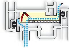
REGEL-air® K - Fensterfalz-Lüfter für Kunststoff-Fenster
