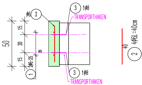
DRAUFSICHT
