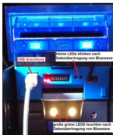
Bild 2: Akzeptorkopf
