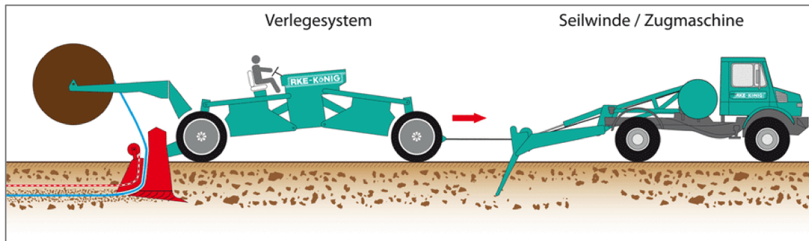
Abbildung 3: Prinzip des Kabelpflug-Verfahrens
