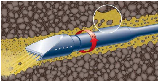
Abbildung 7: Bohrkopf für das Horizontalspülbohr-Verfahren
