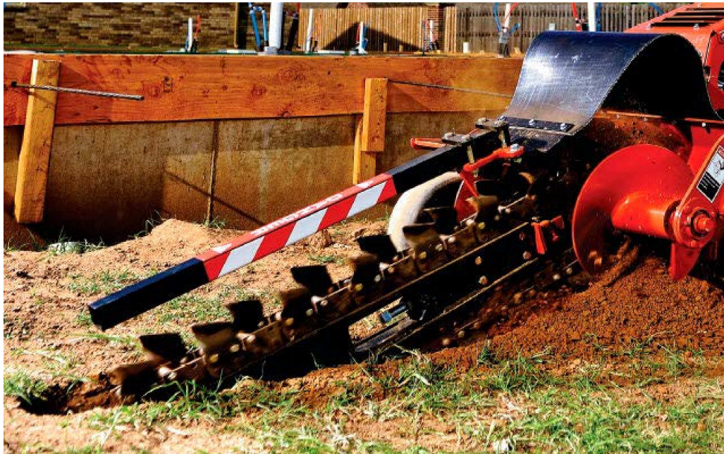
Abbildung 10: Fräs-Verfahren
