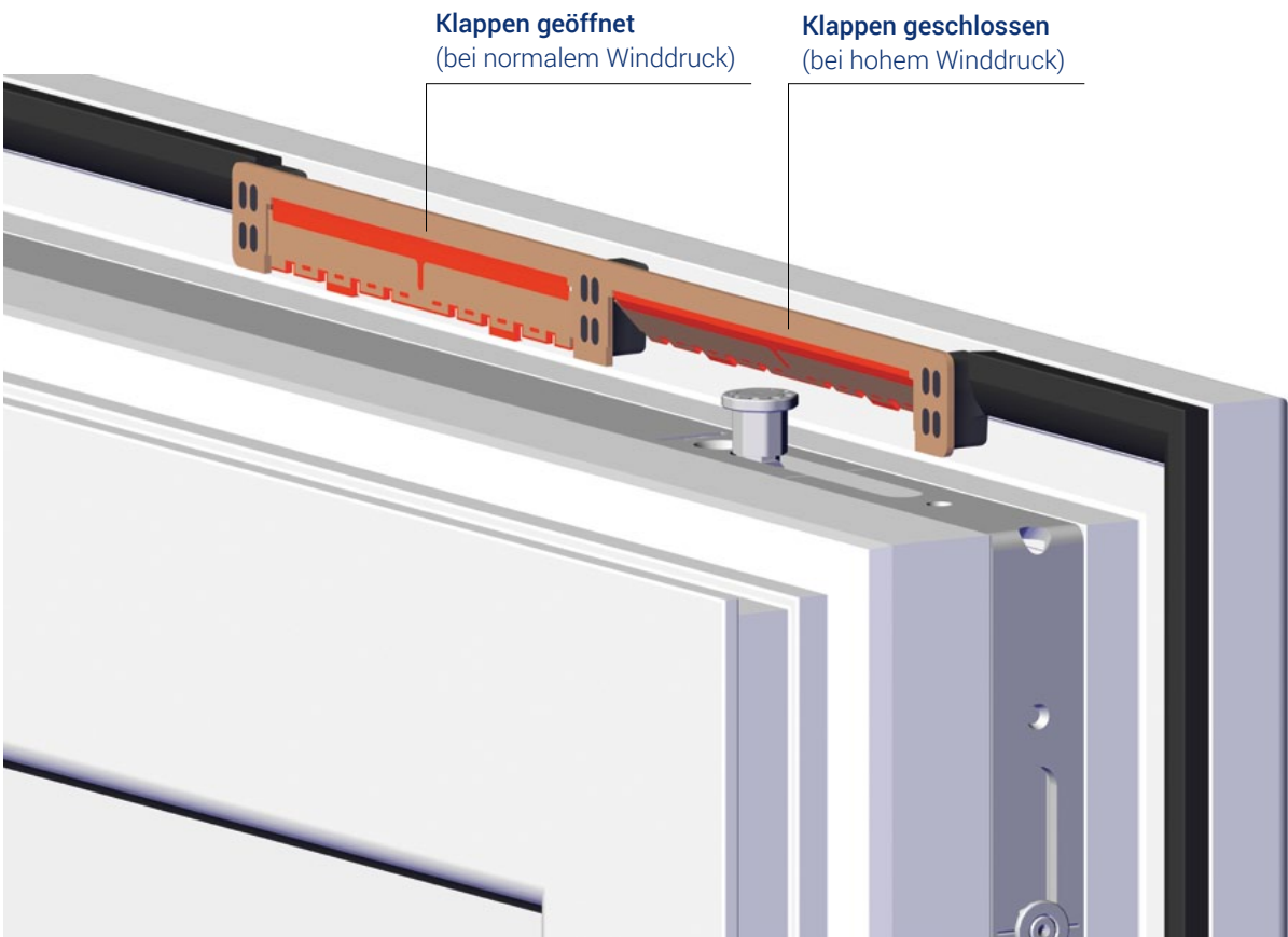
Die unterschiedlichen Klappenzustände dienen der Veranschaulichung. In der Realität öffnen und schließen beide Klappen gleichzeitig.
