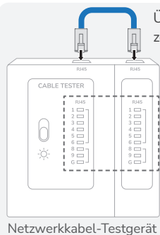
Netzwerk-Kabel-Testgerät
