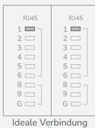
Ideale Verdrahtung
