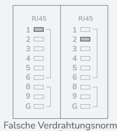
Falsche Verdrahtungsnorm
