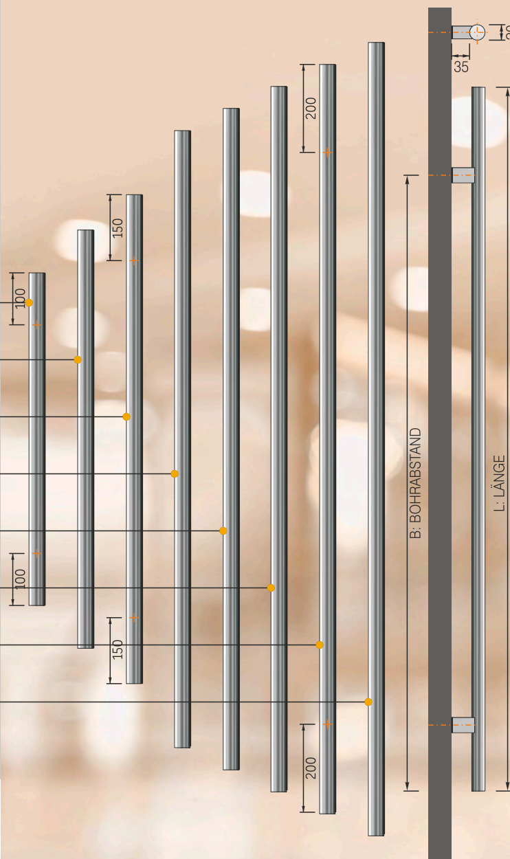
Stoßgriff Edelstahl matt
