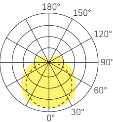
LICHTVERTEILUNGSKURVE
