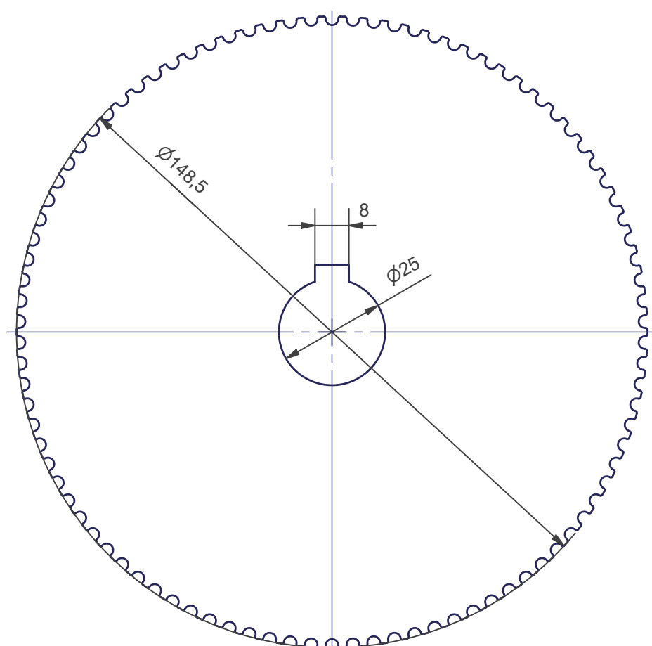
Zahnriemenscheibe 40-1801-002 (04-014-04)
