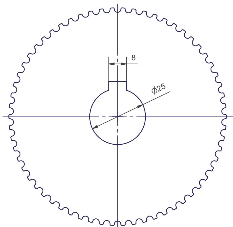
Zahnriemenscheibe 40-1801-001 (04-009-04)
