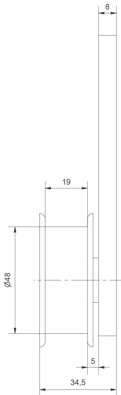
BGR Umlenkrad 110 V2A 40-3100-101
