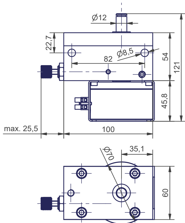
Z03-186-18_BGR2 Feststellvorrichtung
