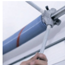
Spannstäbe
