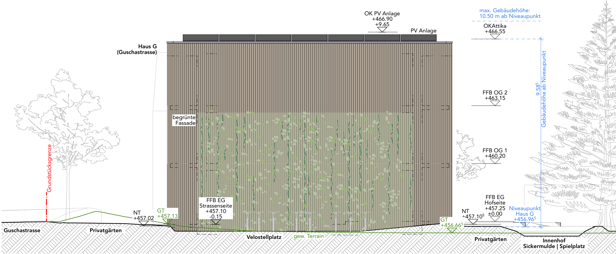
Ansicht Süd | Haus G Stirnseite M 1:100
