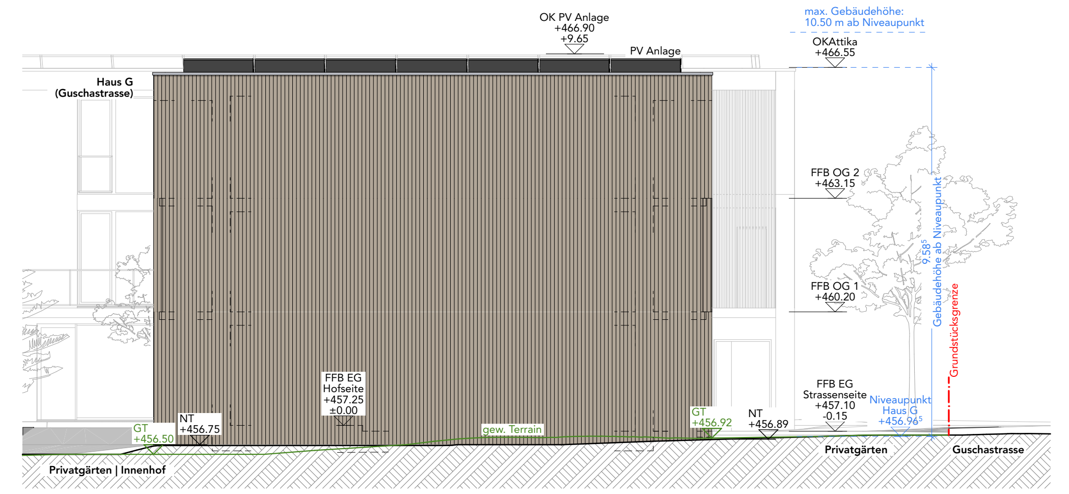
Ansicht Nord | Haus G Stirnseite M 1:100
