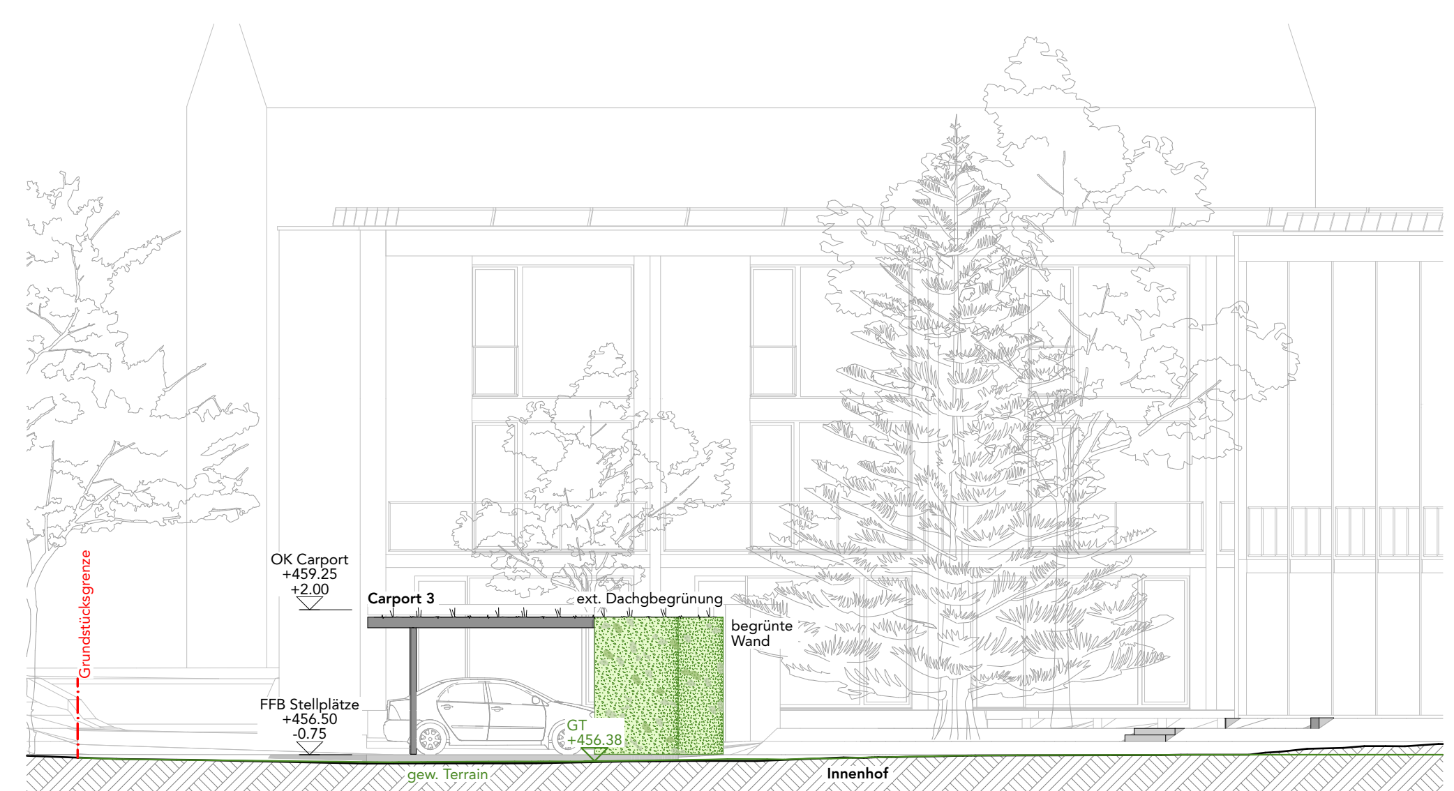
Ansicht Nord | Carport 3 M 1:100
