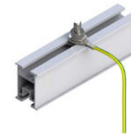
Befestigung des Erdungdrahts mittels Hammerkopfschraube
